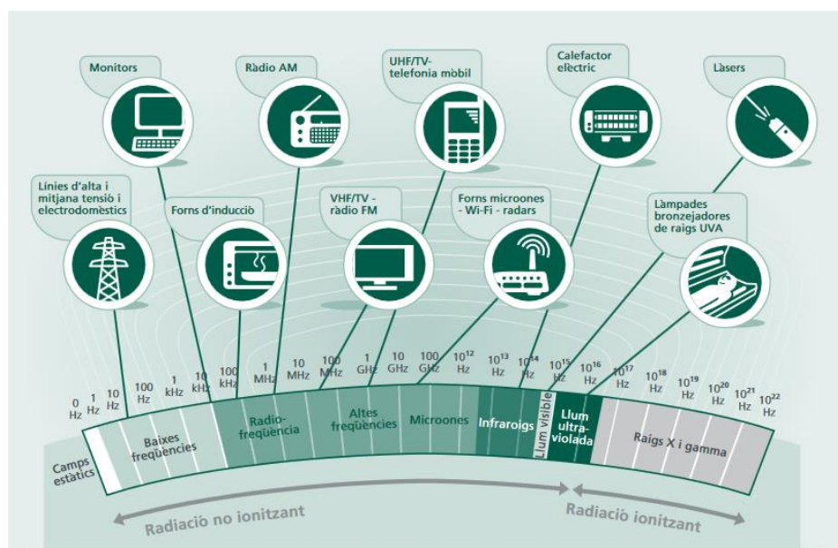
Figura 1. L'espectre electromagnètic
