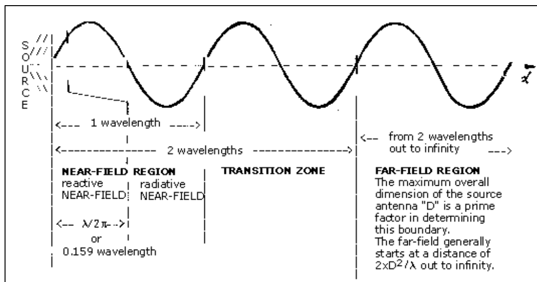
Figura 2. Regions de camp electromagnètic segons la distància de la font
